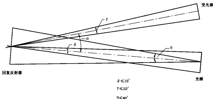
图3 孔径张角与光源发散角
