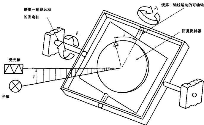
图 2 试样角度旋转系统
