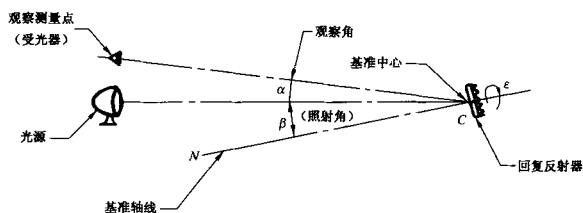
图 1 光度测试原理图
